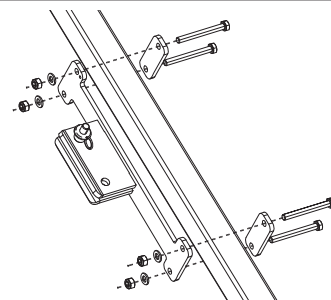
Figura 3 - Instalação do suporte de montagem na SRL
