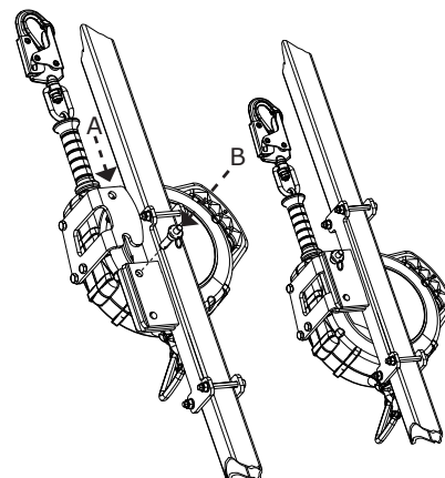
Afbeelding 4 - SRL monteren op verbingsbeugel Protecta Tripod
