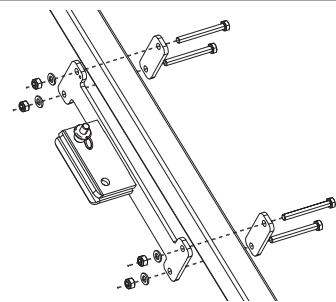
Figur 3 - Montera fäste 3590497 på SRL:en
