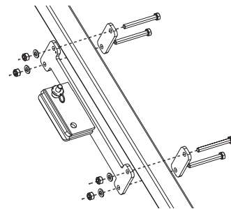
Rys. 3 - Mocowanie wspornika mocującego na urządzeniu samohamownym
