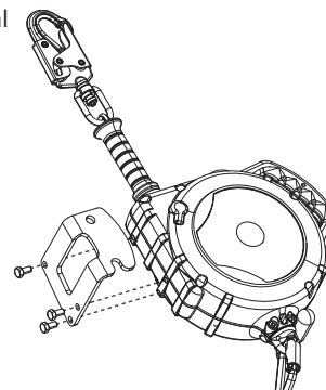
Obrázek 4 - Nainstalujte SRL na párovou podpěru trojnožky Protecta Tripod
