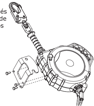
Figura 4: Instalación de las SRL en el soporte de ensamble del trípode Protecta
