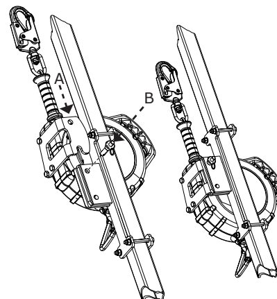
Figura 4 - Montare i cavi SRL sul supporto del treppiede Protecta
