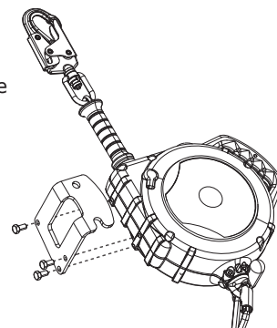
Figur 4 - Montere SRL på festebraketten for Protecta trefot
