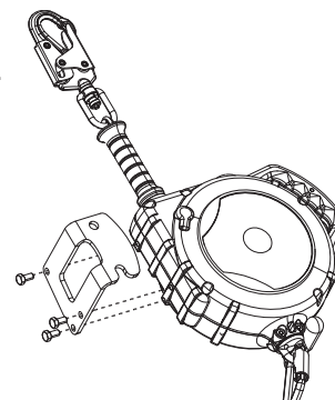
Figura 4 - Montagem da SRL no gancho correspondente do tripé Protecta
