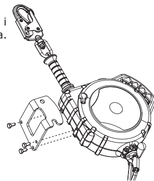
Figur 4 - Montera SRL:en på Protecta-trefotens parningsram
