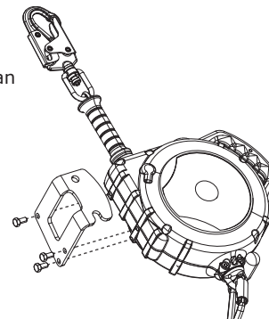
Afbeelding 4 - SRL monteren op verbingsbeugel Protecta Tripod
