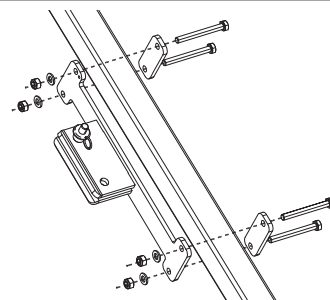
Obrázek 3 - Nainstalujte montážní podpěru na SRL
