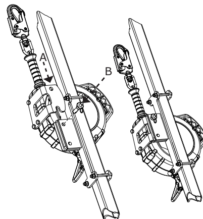
Figure 4 - Installation du dispositif SRL sur le support compatible du trépied Protecta
