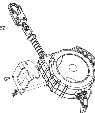
Figure 4 - Installation du dispositif SRL sur le support compatible du trépied Protecta
