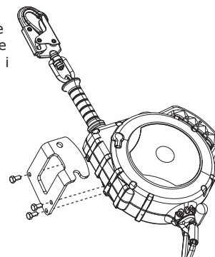
Figura 4 - Montare i cavi SRL sul supporto del treppiede Protecta
